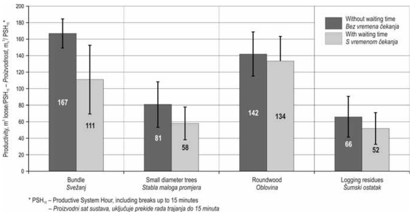
Fig. 6 Chipper productivity in relation to various raw material options with and without operational delays Slika 6. Proizvodnost iverača u ovisnosti o različitim izvorima drvnoga materijala, s prekidom rada i bez prekida
