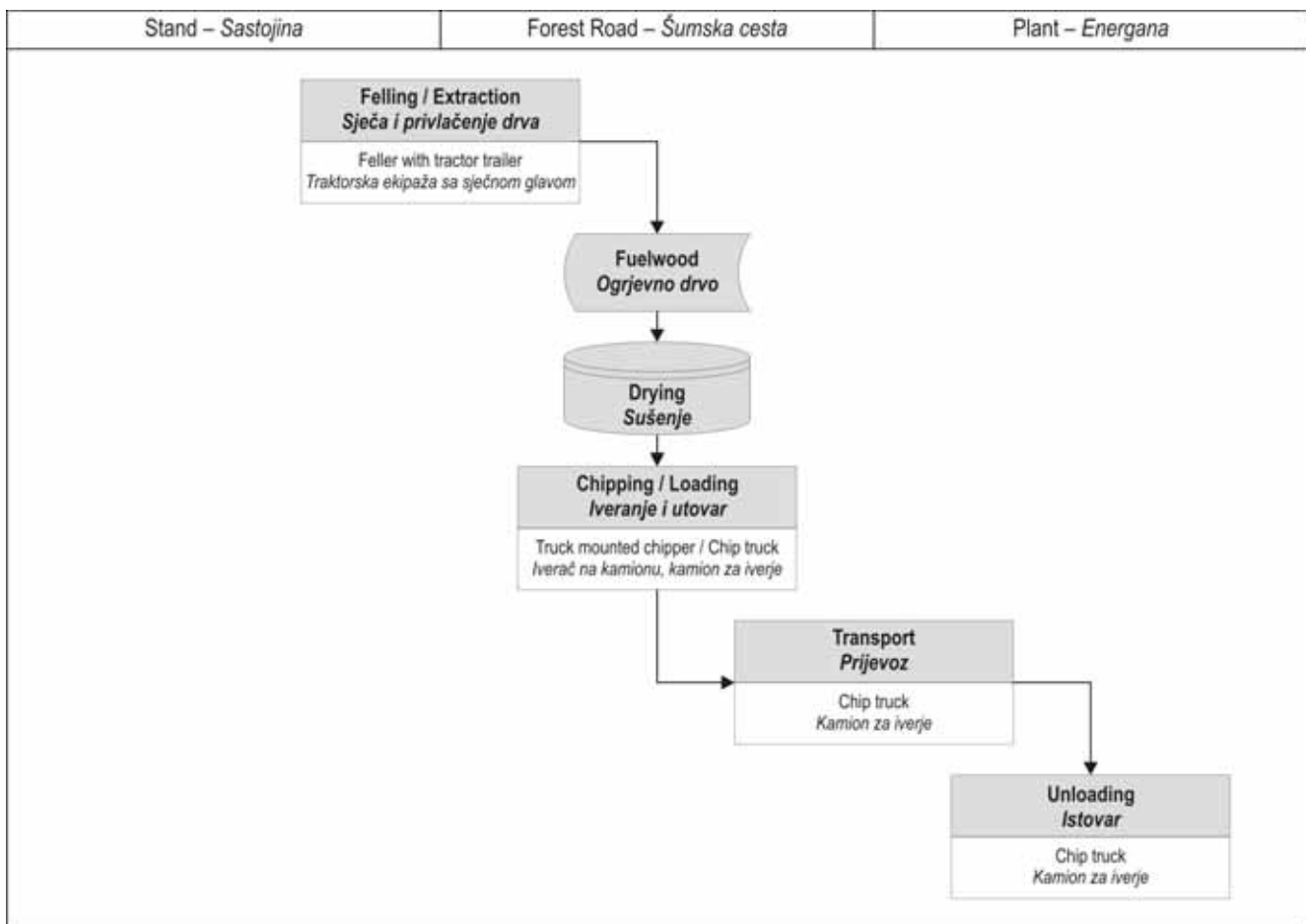
Fig. 5 Utilization of energy wood with shears and tractor trailer in whole-tree extraction; direct chipping into chip trucks Slika 5. Korištenje drva za energiju pri stablovnoj metodi izradbe pri radu traktorske ekipaže sa sječnom glavom, neposredno iveranje u kamione za iverje
